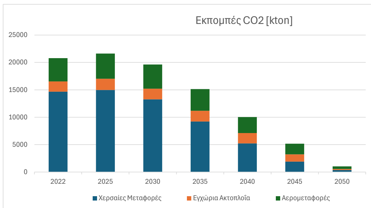
Σχήμα 55 Εκτιμώμενες εκπομπές ανά κλάδο μεταφορών, ανά 5-ετία για την περίοδο 2025-2050.
