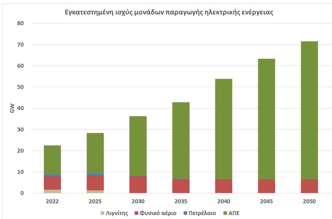
Σχήμα 35 Εξέλιξη της εγκατεστημένης ισχύος των μονάδων ηλεκτροπαραγωγής έως το έτος 2050.
