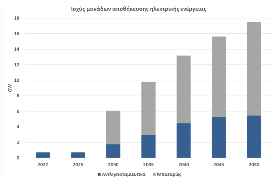
Σχήμα 40 Εξέλιξη της ισχύος μονάδων αποθήκευσης ηλεκτρικής ενέργειας έως το έτος 2050.
