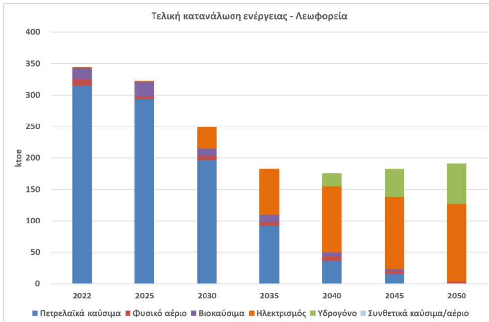
Σχήμα 51 Εξέλιξη τελικής κατανάλωσης ενέργειας στα λεωφορεία έως το έτος 2050.
