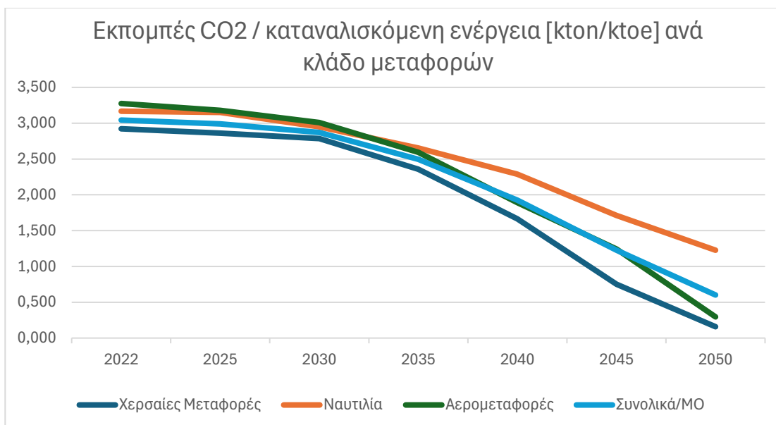
Σχήμα 8 Εξέλιξη δείκτη εκπομπών CO 2 ανά μονάδα καταναλισκόμενης ενέργειας (kton CO 2 /ktoe), μέσος όρος τομεά και ανά κλάδο μεταφορών.
