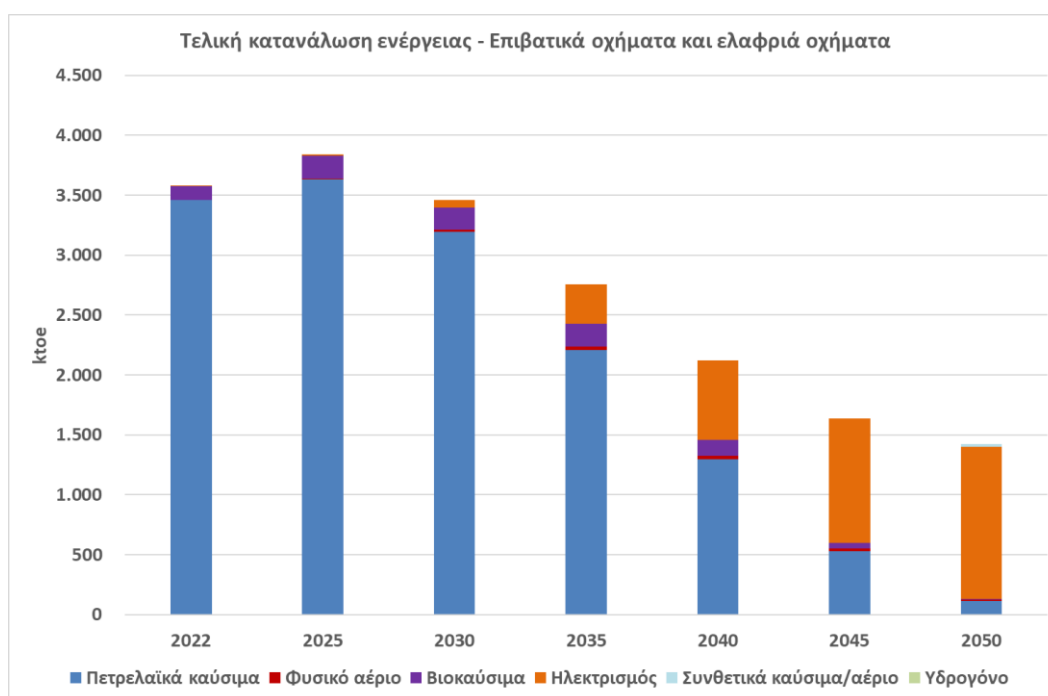
Σχήμα 49 Εξέλιξη τελικής κατανάλωσης ενέργειας στα επιβατικά και ελαφριά οχήματα έως το έτος 2050.
