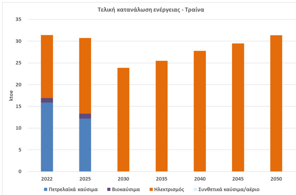
Σχήμα 52 Εξέλιξη τελικής κατανάλωσης ενέργειας στα τραίνα έως το έτος 2050.
