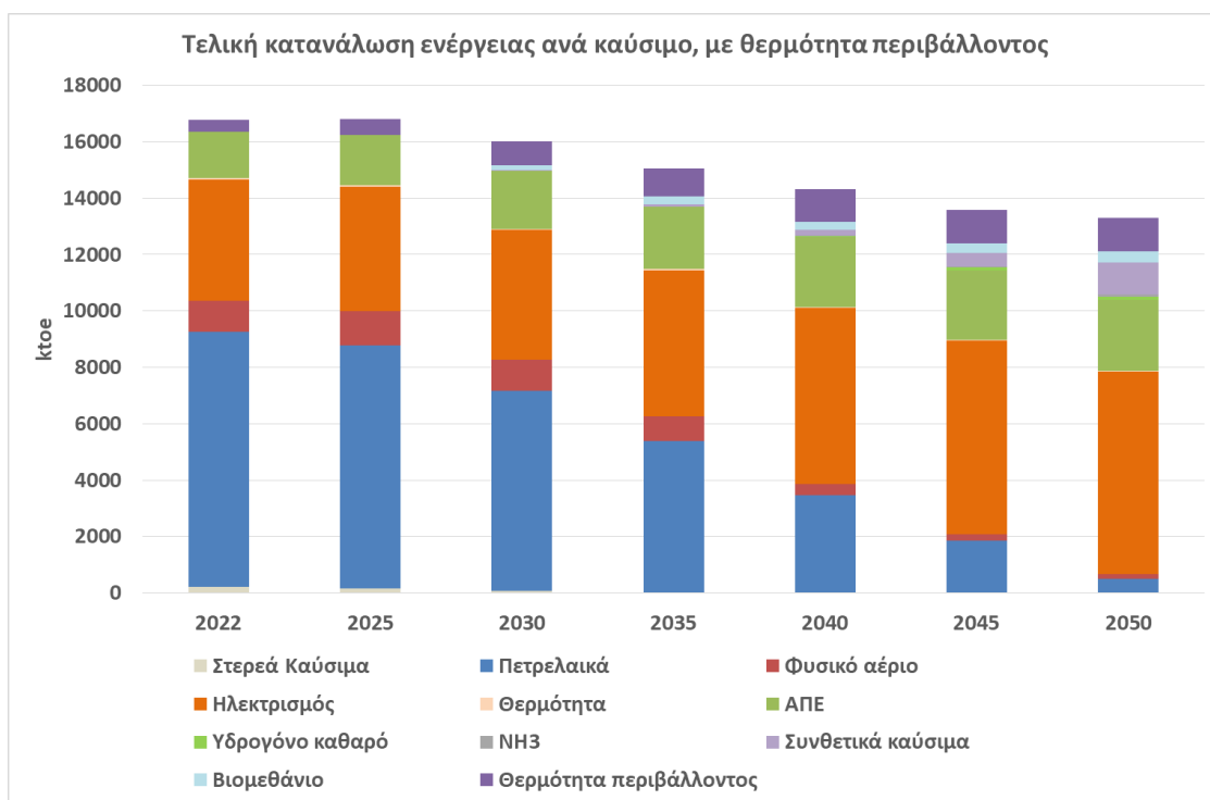
Σχήμα 30 Εξέλιξη των μεριδίων καυσίμων τελικής κατανάλωσης ενέργειας έως το έτος 2050.
