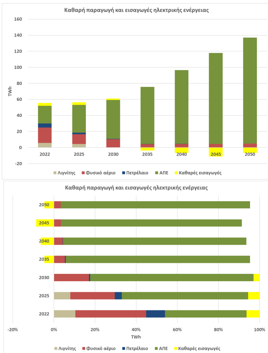
Σχήμα 37 Εξέλιξη της καθαρής παραγωγής και των εισαγωγών ηλεκτρικής ενέργειας έως το έτος 2050, (σε TWh και ως ποσοστό).
