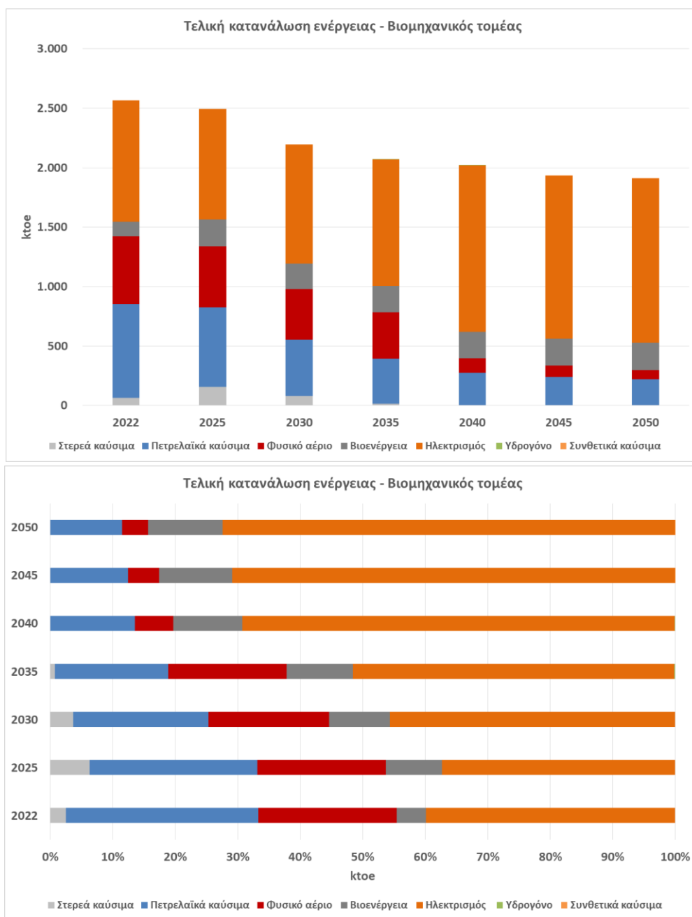
Σχήμα 56 Εξέλιξη τελικής κατανάλωσης ενέργειας στον τομέα της βιομηχανίας έως το έτος 2050.
