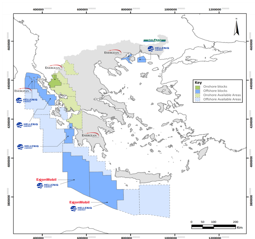
Εικόνα 12 Οικόπεδα ερευνών για υδρογονάνθρακες.
