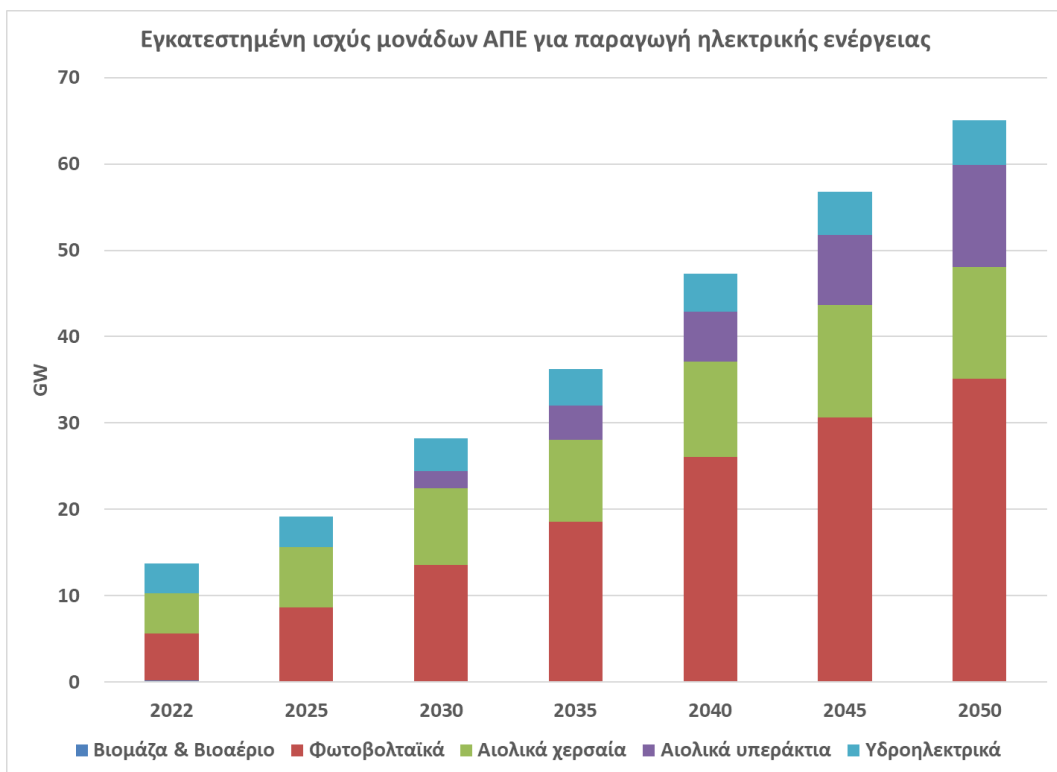
Σχήμα 36 Εξέλιξη της εγκατεστημένης ισχύος ΑΠΕ για Ηλεκτροπαραγωγή έως το έτος 2050.
