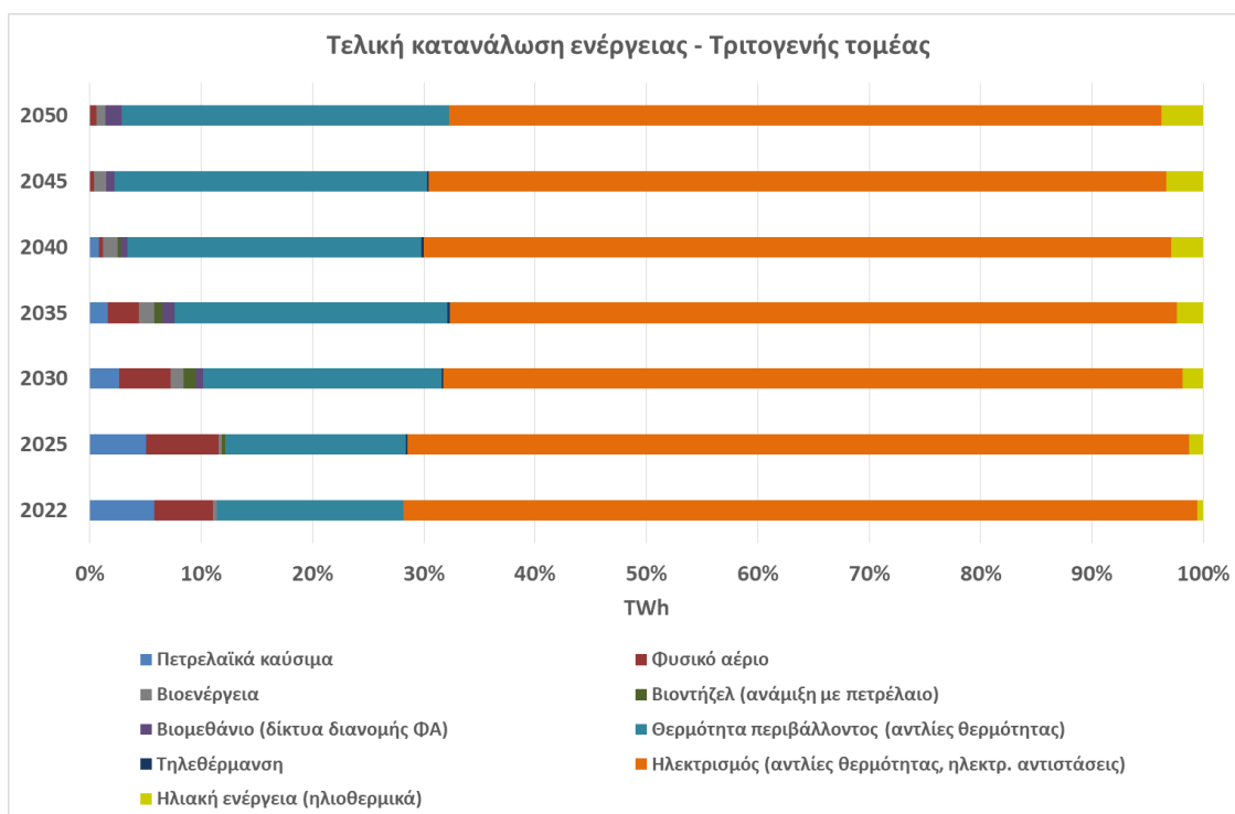
Σχήμα 46 Εξέλιξη τελικής κατανάλωσης ενέργειας στον τριτογενή τομέα έως το έτος 2050.
