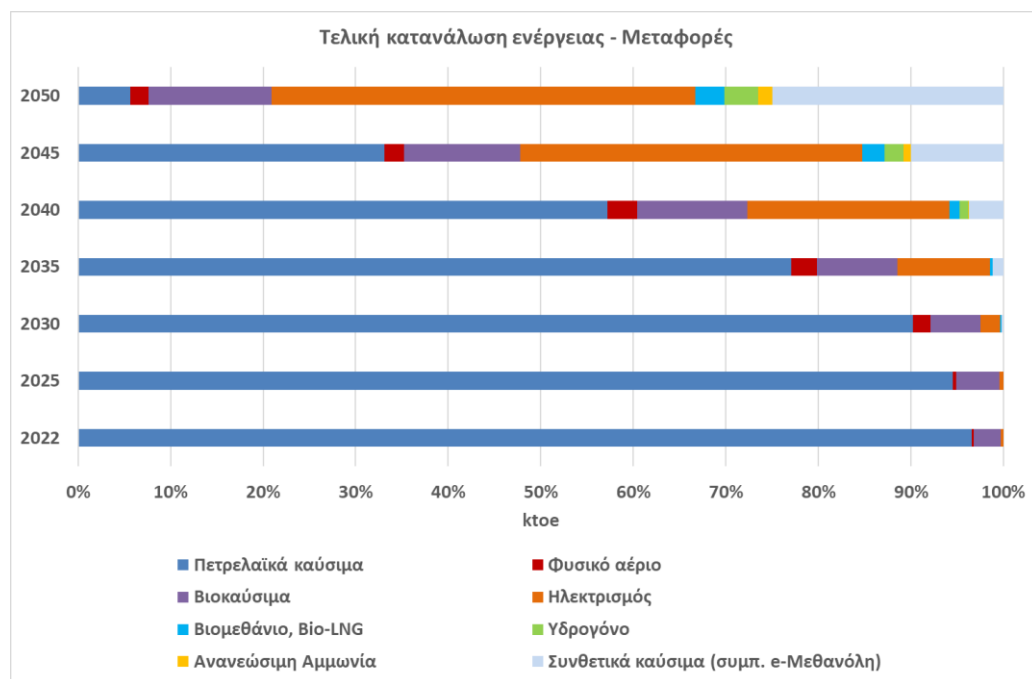
Σχήμα 47 Εξέλιξη τελικής κατανάλωσης ενέργειας στον τομέα των μεταφορών έως το έτος 2050.
