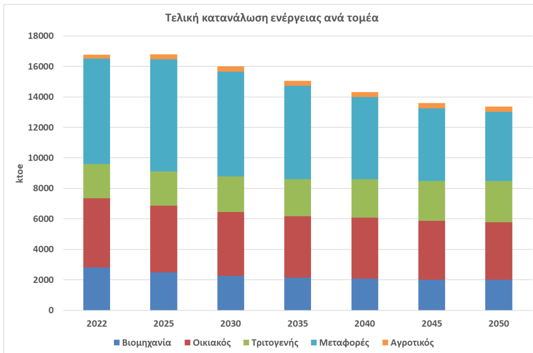
Σχήμα-ΕΣ 12 Εξέλιξη τελικής κατανάλωσης ενέργειας ανά τομέα έως το έτος 2050.
