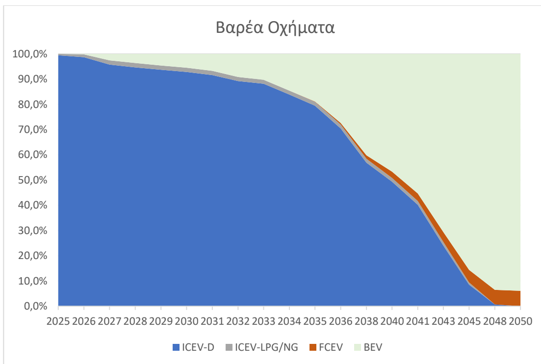
Σχήμα 10 Εκτιμώμενη εξέλιξη στόλου βαρέων οχημάτων ως ποσοστό (%) κάθε τύπου κινητήρα (καυσίμου) επί του συνόλου, για την περίοδο 2025-2050.
