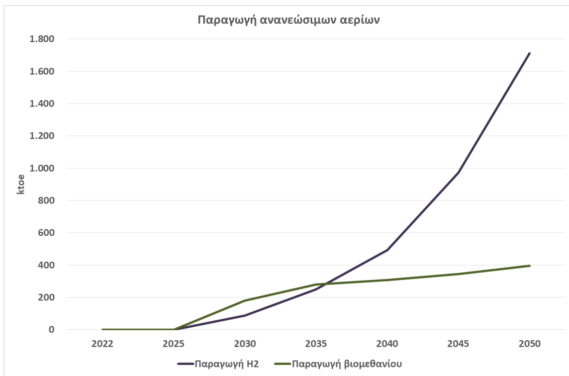
Σχήμα-ΕΣ 11 Εξέλιξη παραγωγής ανανεώσιμων αερίων έως το έτος 2050.
