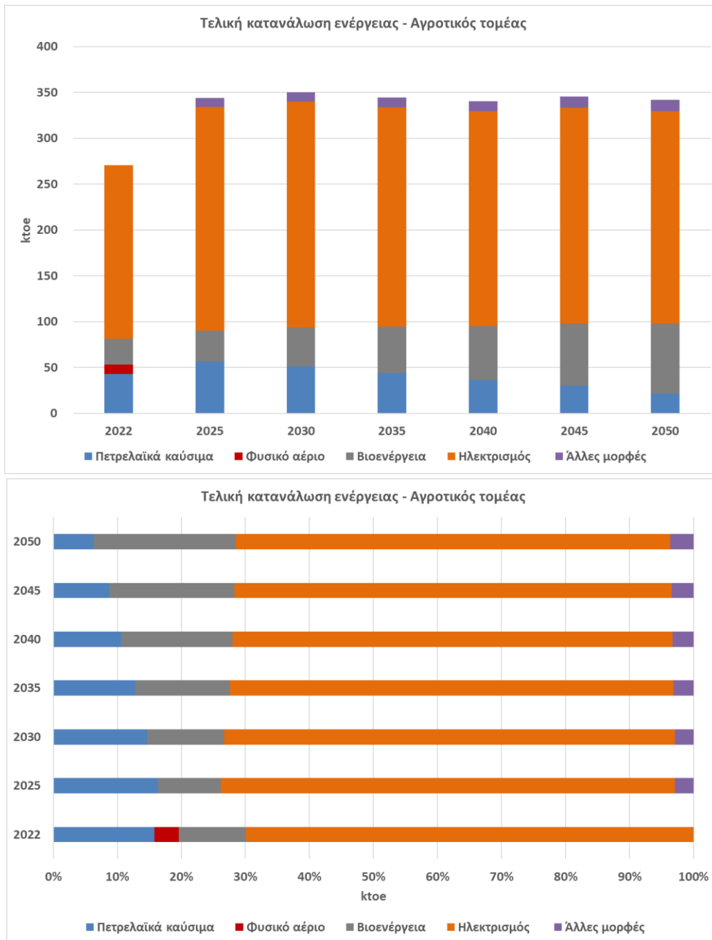
Σχήμα 57 Εξέλιξη τελικής κατανάλωσης ενέργειας στον αγροτικό τομέα έως το έτος 2050.
