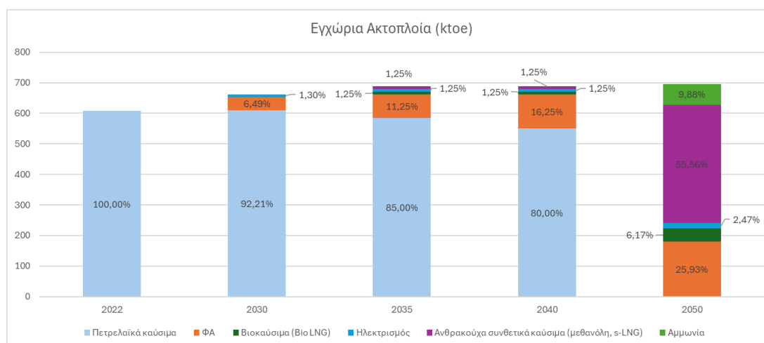
Σχήμα-ΕΣ 16 Κατανάλωση ενέργειας στην εγχώρια ακτοπλοΐα ανά τύπο καυσίμου (κτοε).
