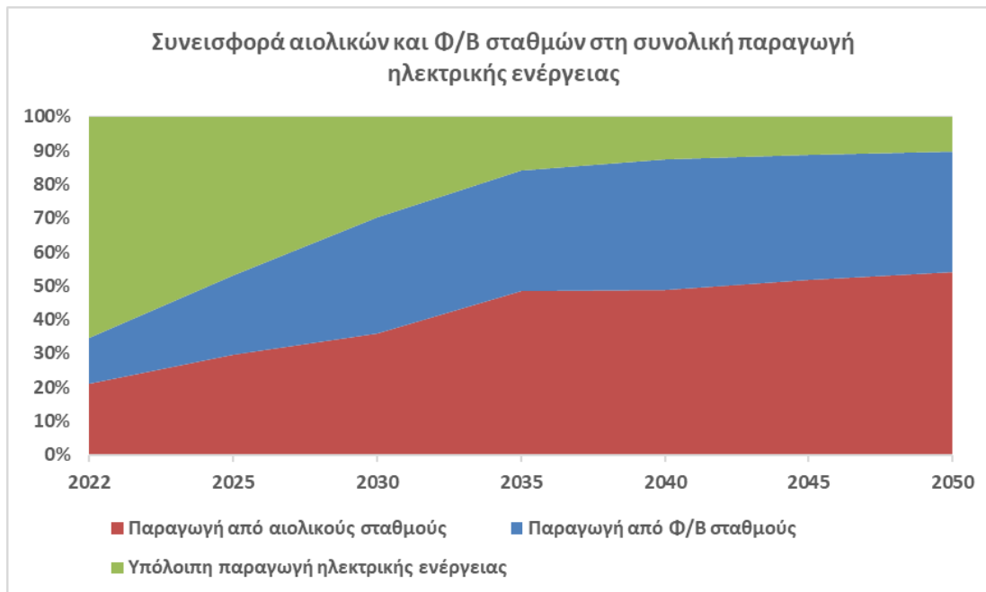
Σχήμα 39 Μερίδιο ηλεκτροπαραγωγής από αιολικούς και φωτοβολταϊκούς σταθμούς στο σύνολο της διάθεσης ηλεκτρικής ενέργειας έως το έτος 2050.
