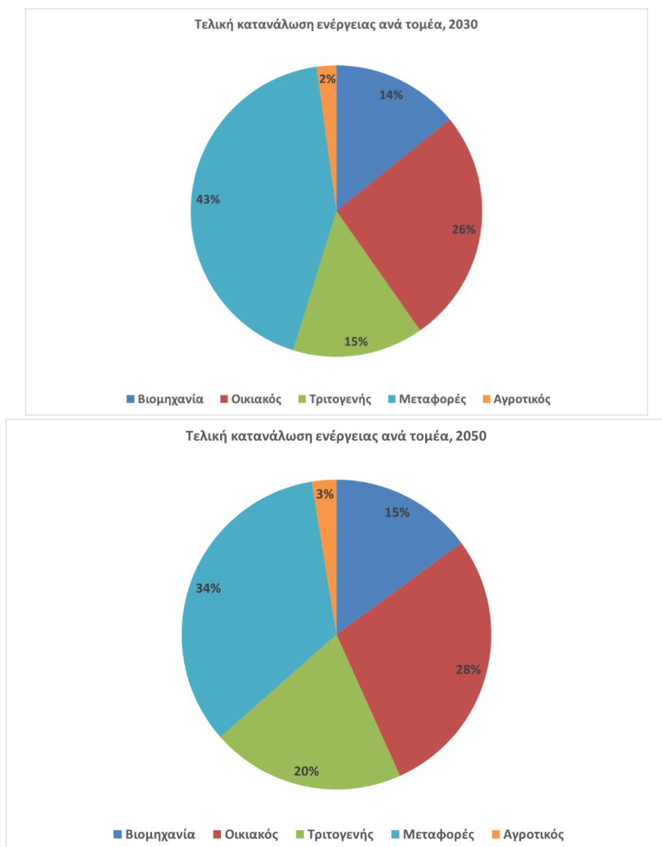
Σχήμα 43 Εξέλιξη τελικής κατανάλωσης ενέργειας ανά τομέα σε ποσοστιαία βάση τα έτη 2030 και 2050.
