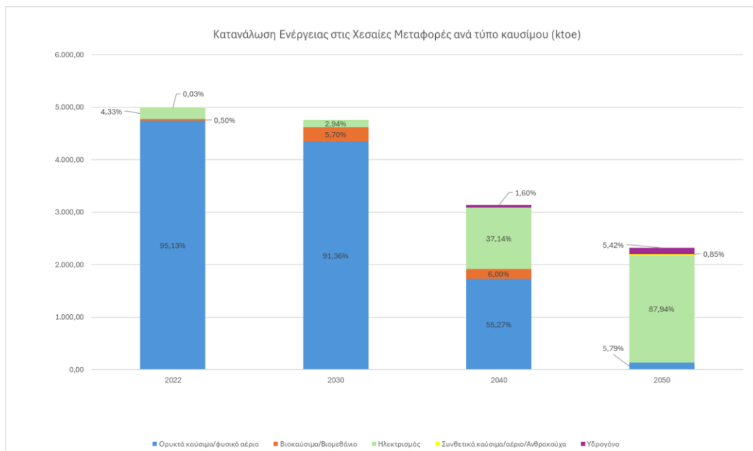
Σχήμα-ΕΣ 14 Κατανάλωση ενέργειας στις χερσαίες μεταφορές ανά τύπο καυσίμου (ktoe).
