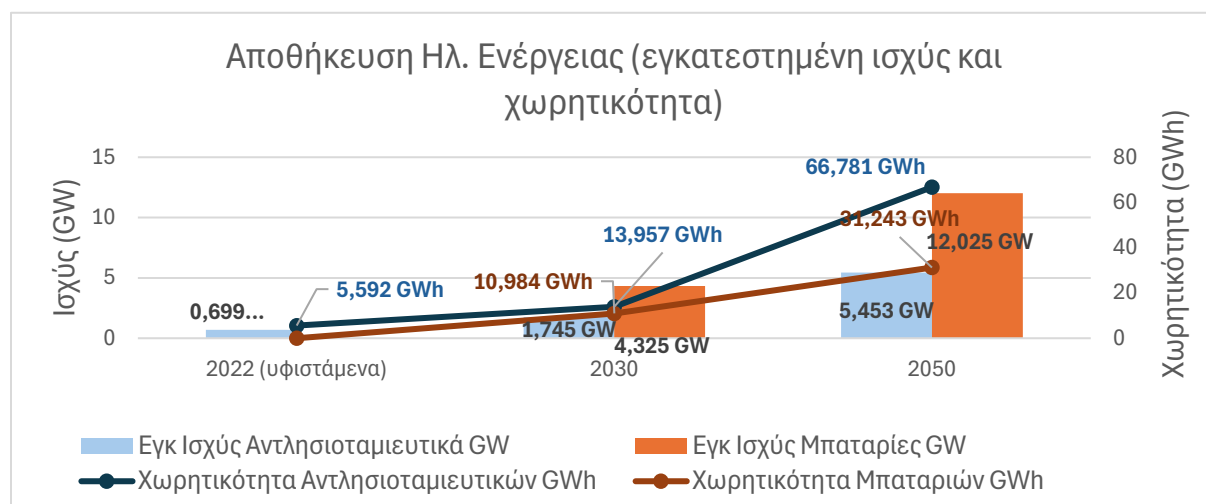
Σχήμα-ΕΣ 8 Εξέλιξη αποθήκευσης ηλεκτρικής ενέργειας (ισχύς και χωρητικότητα μονάδων) για τα έτη 2022 (ιστορικά), 2030 και 2050.
