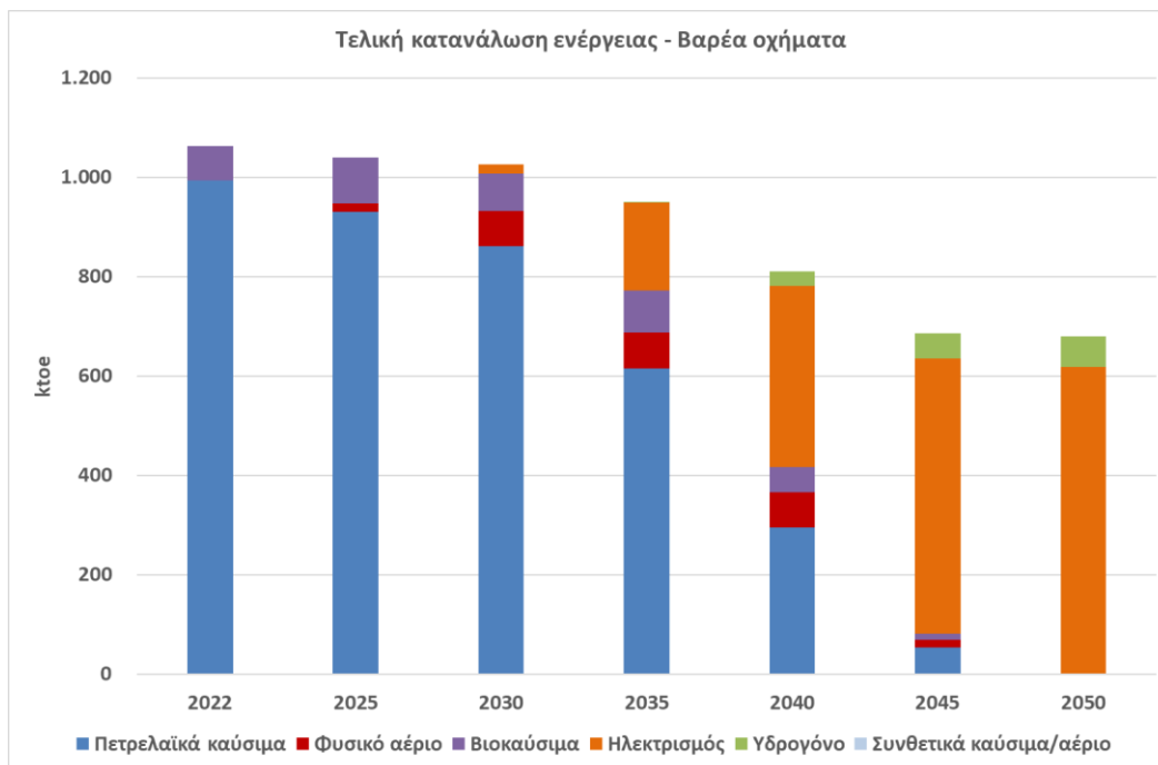
Σχήμα 50 Εξέλιξη τελικής κατανάλωσης ενέργειας στα βαρέα οχήματα έως το έτος 2050.
