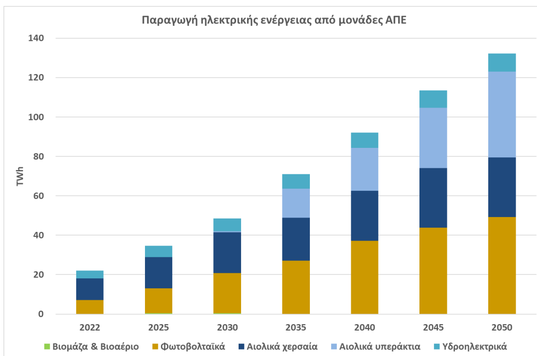
Σχήμα 38 Εξέλιξη της ηλεκτροπαραγωγής από ΑΠΕ έως το έτος 2050.
