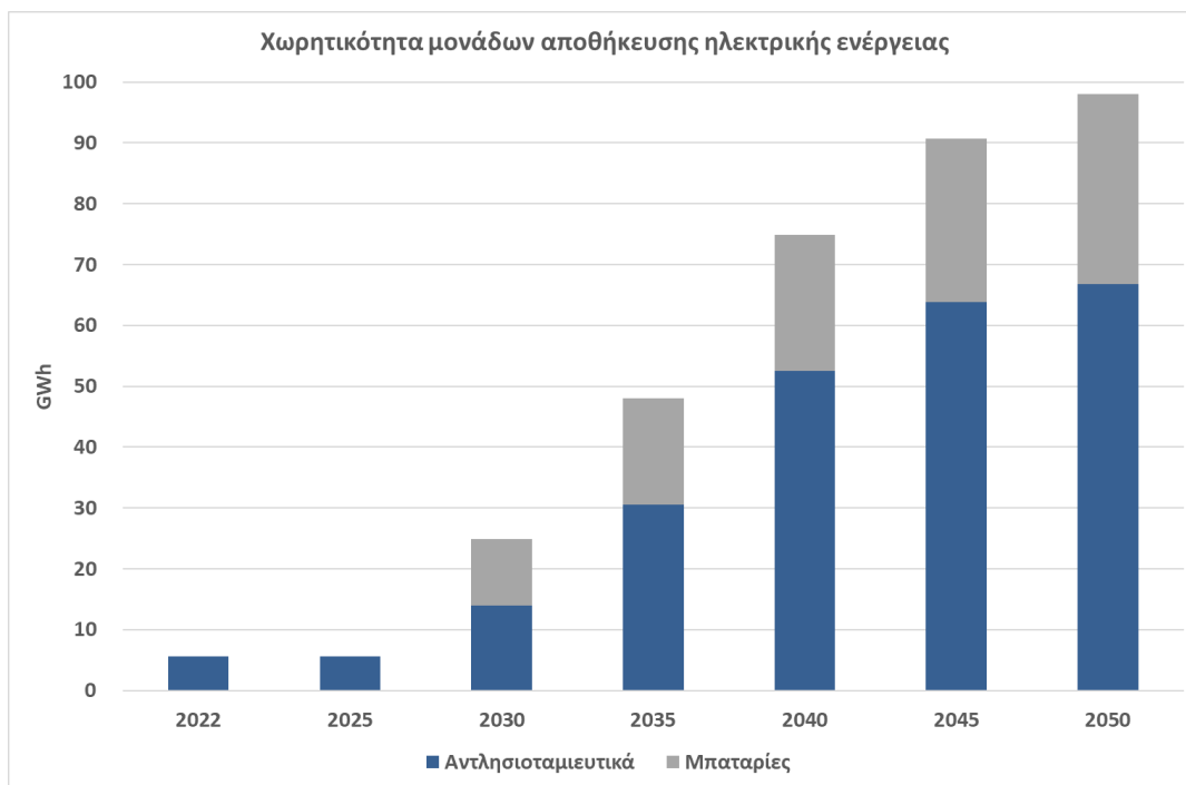
Σχήμα 41 Εξέλιξη της χωρητικότητας μονάδων αποθήκευσης ηλεκτρικής ενέργειας έως το έτος 2050.
