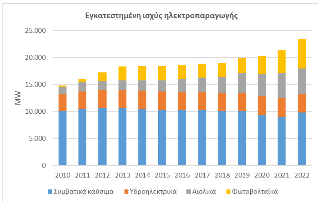
Σχήμα 18 Εγκατεστημένη ισχύς ηλεκτροπαραγωγής για την περίοδο 2010-2022 (Πηγή: Eurostat).
