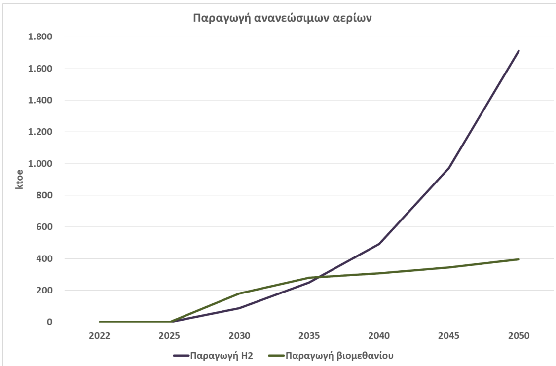
Σχήμα 34 Εξέλιξη παραγωγής ανανεώσιμων αερίων έως το έτος 2050.
