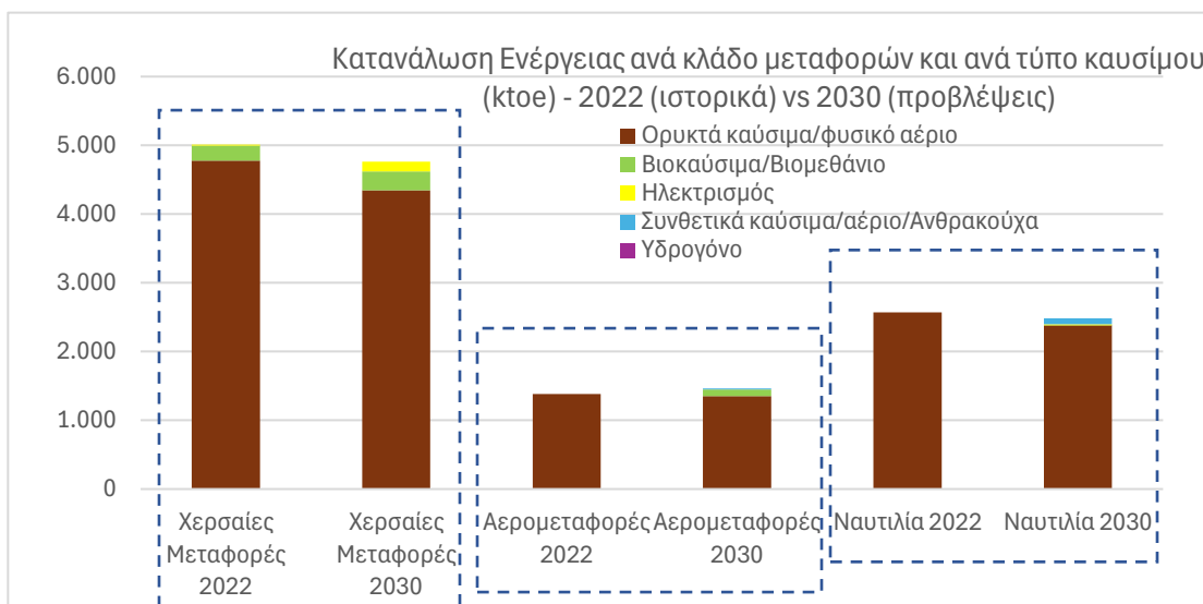
Σχήμα 6 Ενεργειακή κατανάλωση (σε 000 τιπ) ανά κλάδο μεταφορών και τύπο καυσίμου, για τα έτη 2022 (ιστορικά) και το 2030 (προβλέψεις).
