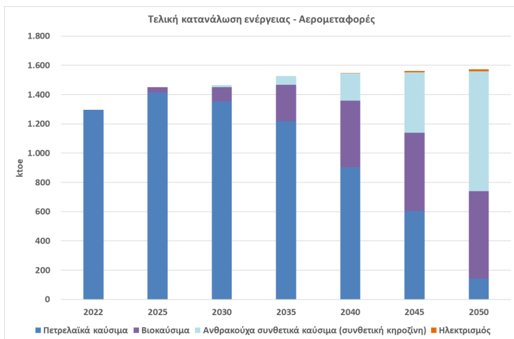
Σχήμα 54 Εξέλιξη τελικής κατανάλωσης ενέργειας στις αερομεταφορές έως το έτος 2050
