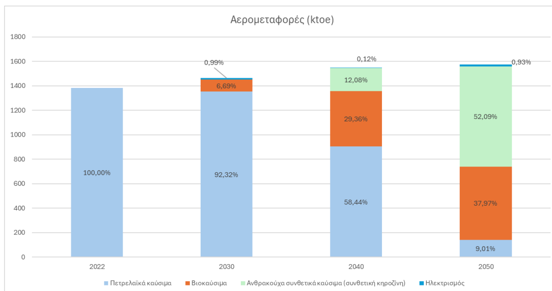
Σχήμα-ΕΣ 15 Κατανάλωση ενέργειας στις αεροπορικές μεταφορές ανά τύπο καυσίμου (κτοε).
