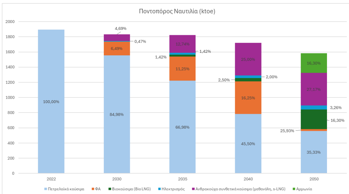
Σχήμα-ΕΣ 17 Κατανάλωση ενέργειας στην ποντοπόρο ναυτιλία ανά τύπο καυσίμου (κτοε).
