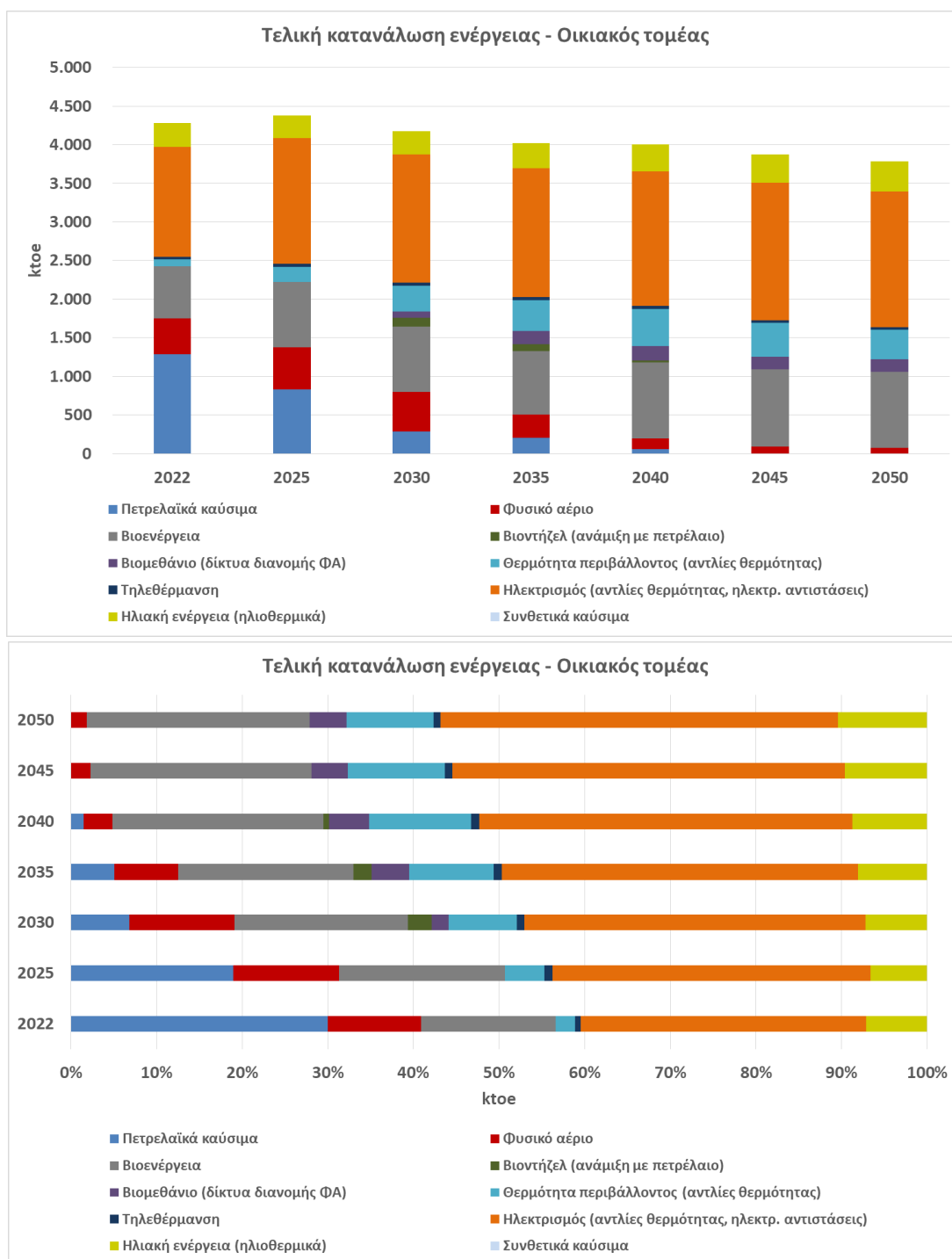
Σχήμα 45 Εξέλιξη τελικής κατανάλωσης ενέργειας στον οικιακό τομέα έως το έτος 2050.
