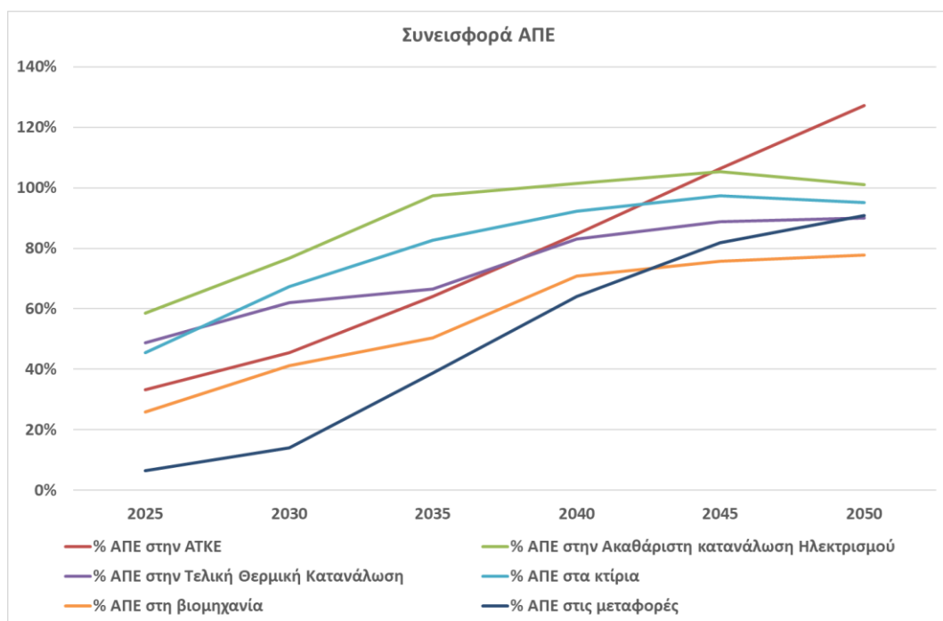
Σχήμα 21 Ειδικά μερίδια συμμετοχής των ΑΠΕ στο εγχώριο ενεργειακό σύστημα στη βάση μεθοδολογίας της Ευρωπαϊκής Ένωσης.
