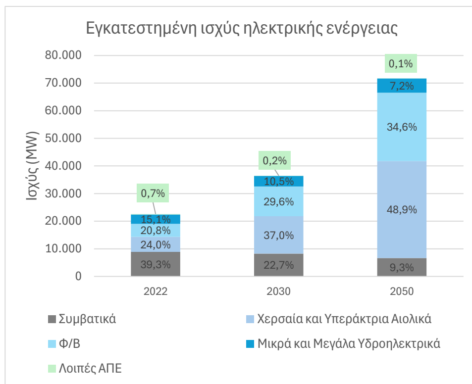
Σχήμα-ΕΣ 7 Εγκατεστημένη ισχύς μονάδων ηλεκτροπαραγωγής, για την περίοδο 2022 (ιστορικά) έως 2050.
