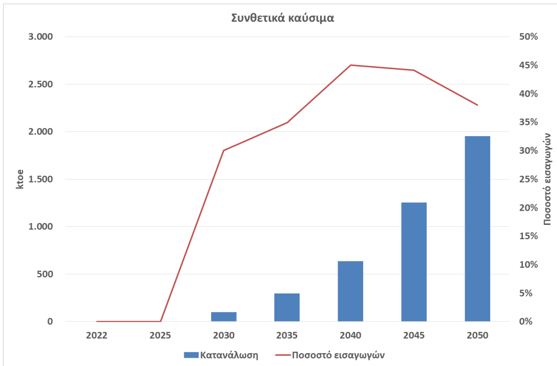
Σχήμα 33 Εξέλιξη κατανάλωσης συνθετικών καυσίμων και ποσοστό εισαγωγών αυτών έως το έτος 2050.
