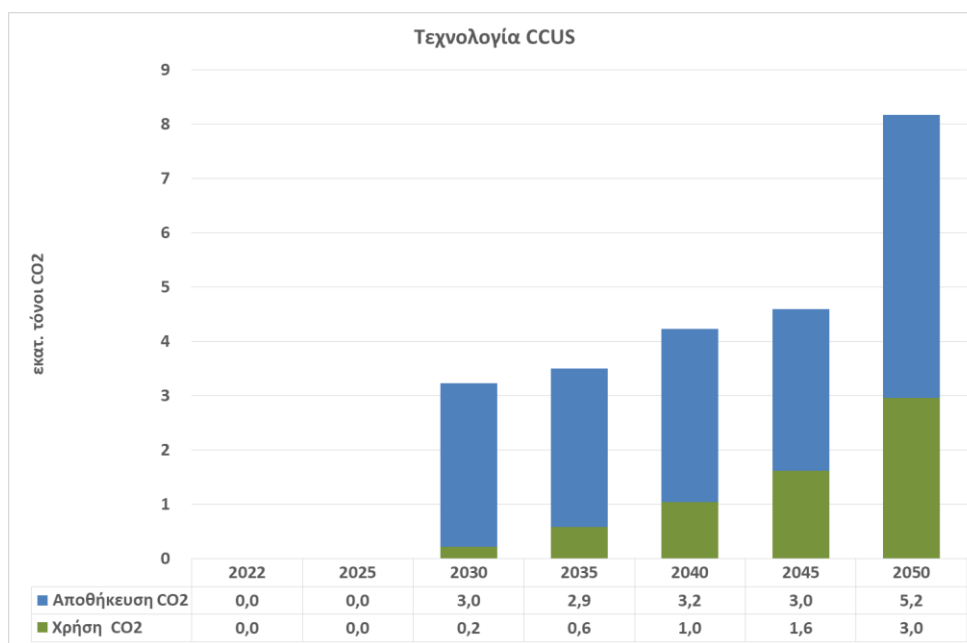
Σχήμα 20 Κάλυψη αναγκών για CCUS έως το έτος 2050.
