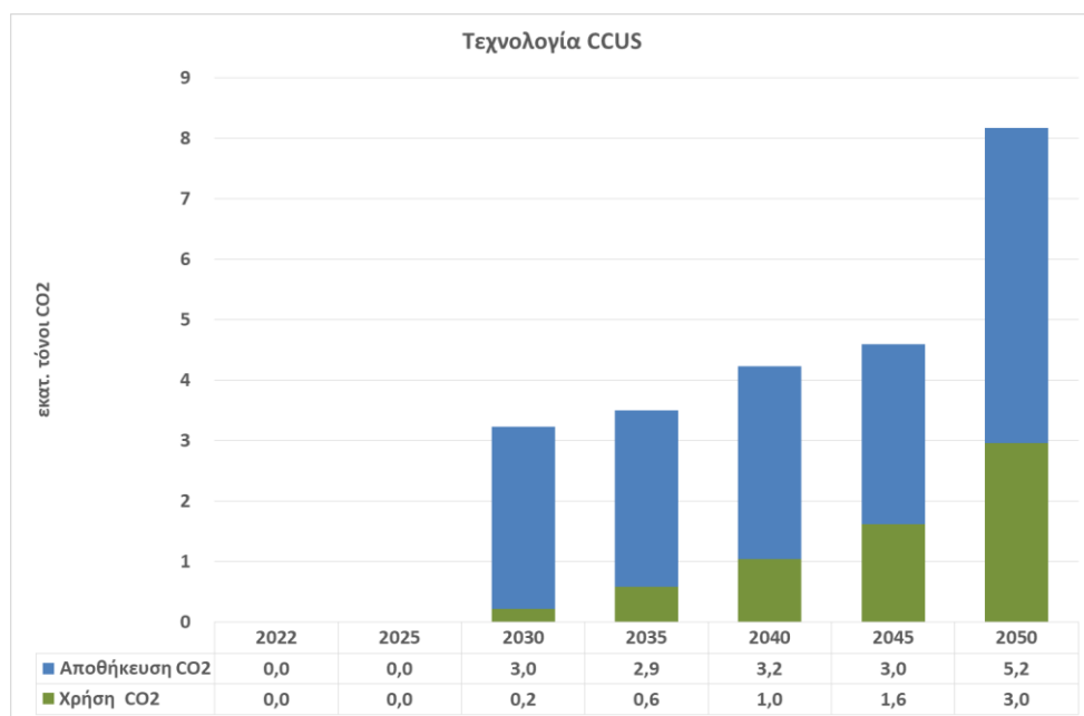
Σχήμα-ΕΣ 10 Κάλυψη αναγκών για δέσμευση και αποθήκευση διοξειδίου του άνθρακα των καυσαερίων (CCUS), έως το έτος 2050.
