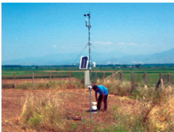
Μέτρηση εδαφικής υγρασίας στο χωράφι (Βαμβάκι)
